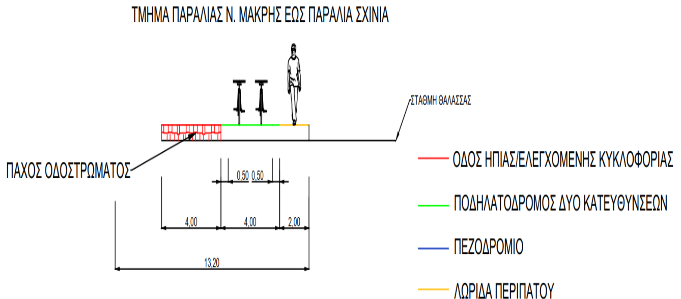
Εικόνα 2: Τυπική Διατομή προτεινόμενων έργων στο Παραλιακό Μέτωπο.
