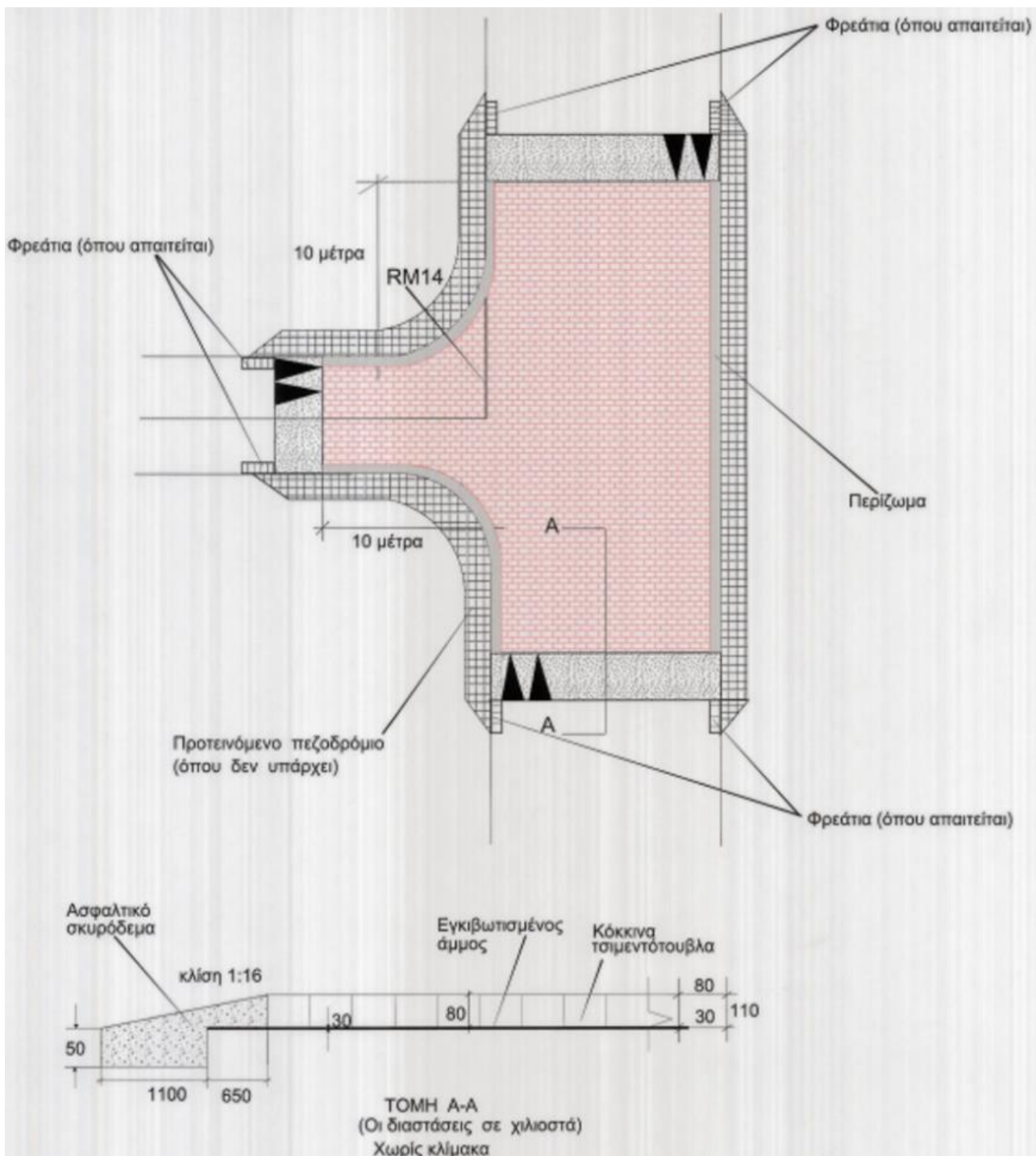
Εικόνα 19: Τυπικό Σχέδιο Υπερυψωμένης Συμβολής (πλατό).
