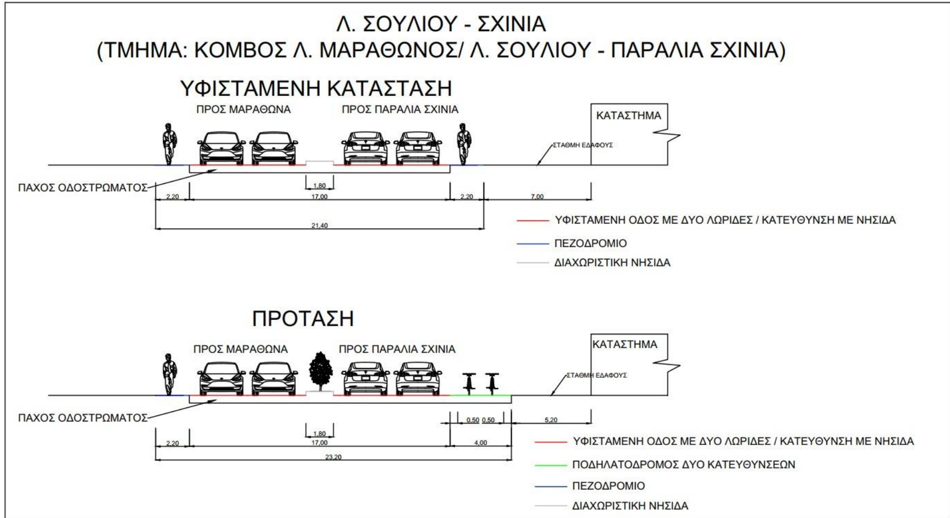
Εικόνα 13: Τυπική Διατομή στη Λεωφ. Σουλίου – Σχινιά.
