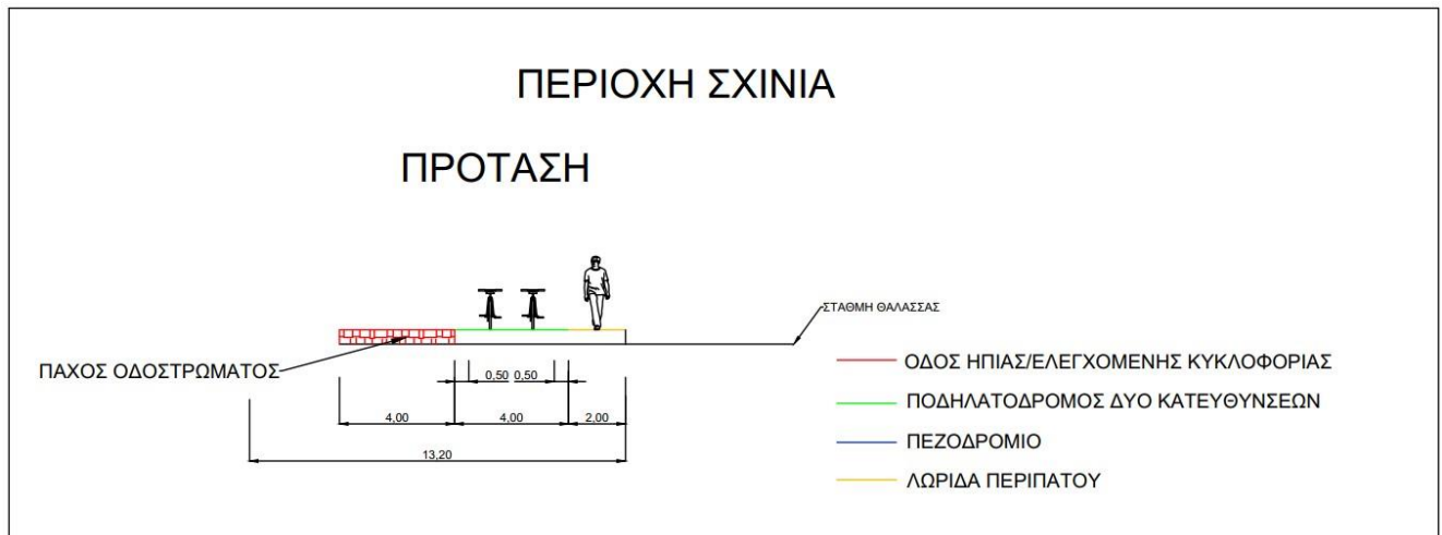
Εικόνα 10: Τυπική διατομή στην περιοχή Σχινιά.
