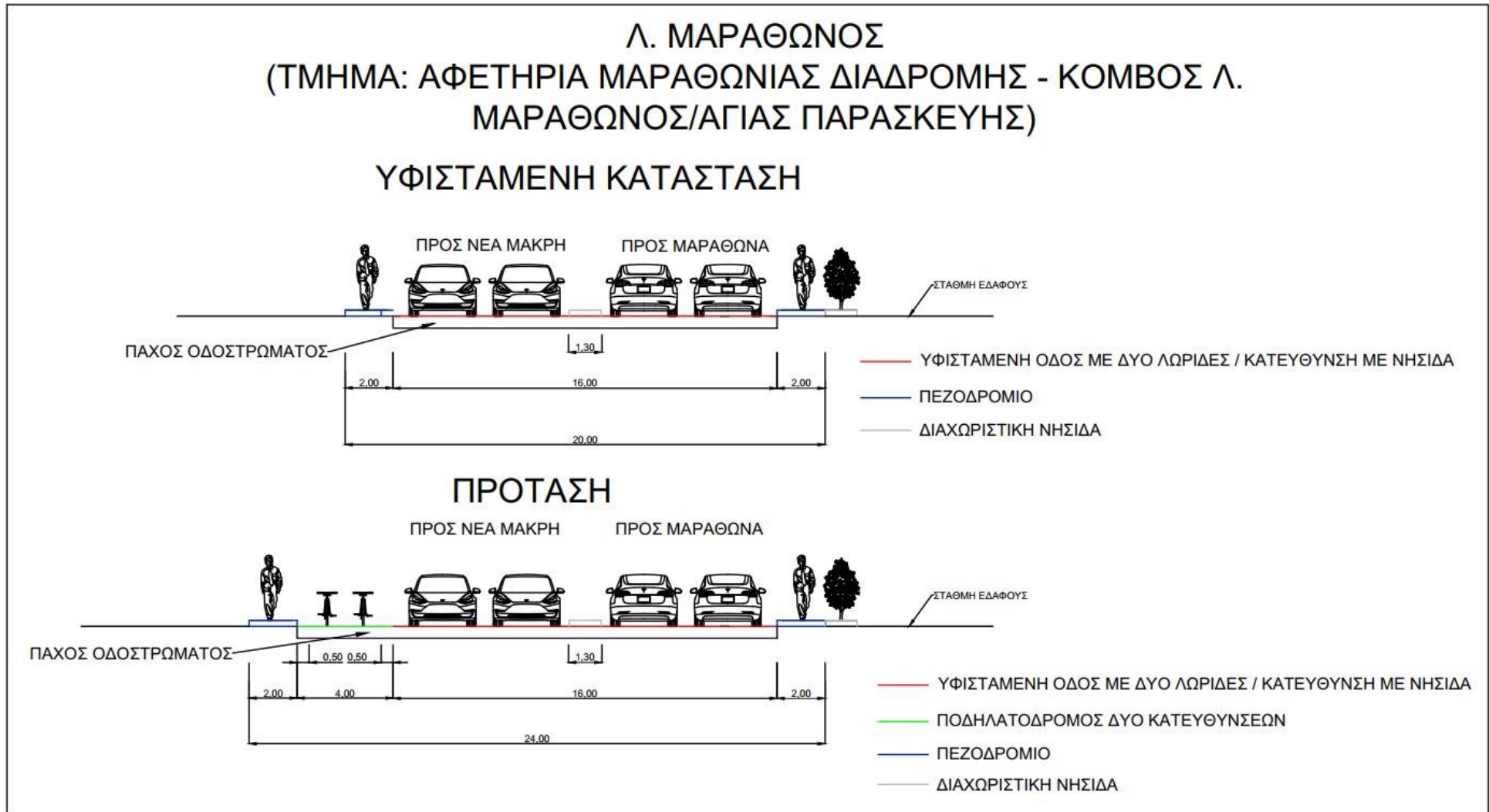
Εικόνα 11: Τυπική Διατομή στη Λεωφ. Μαραθώνος.
