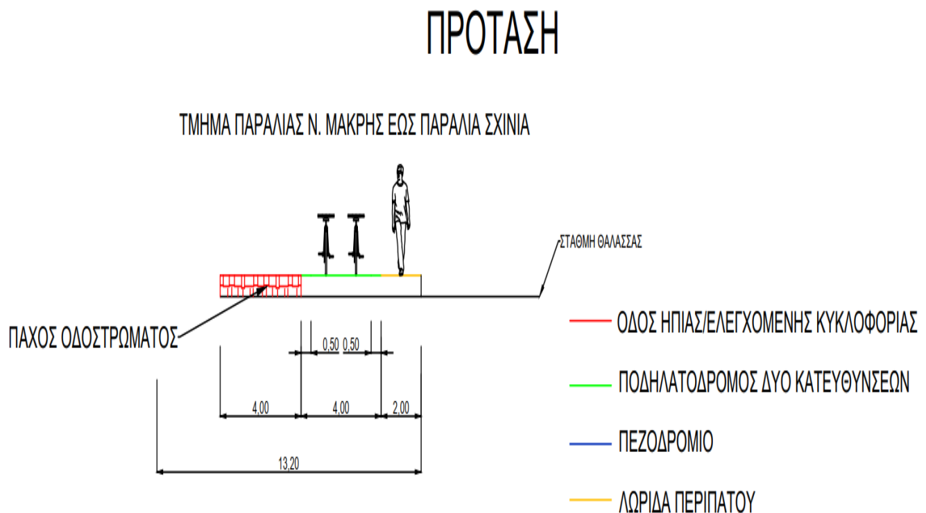
Εικόνα 2: Τυπική Διατομή προτεινόμενων έργων στο Παραλιακό Μέτωπο.
