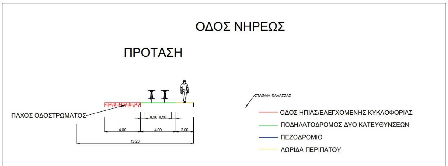
Εικόνα 8: Τυπική Διατομή στην οδό Νηρέως.
