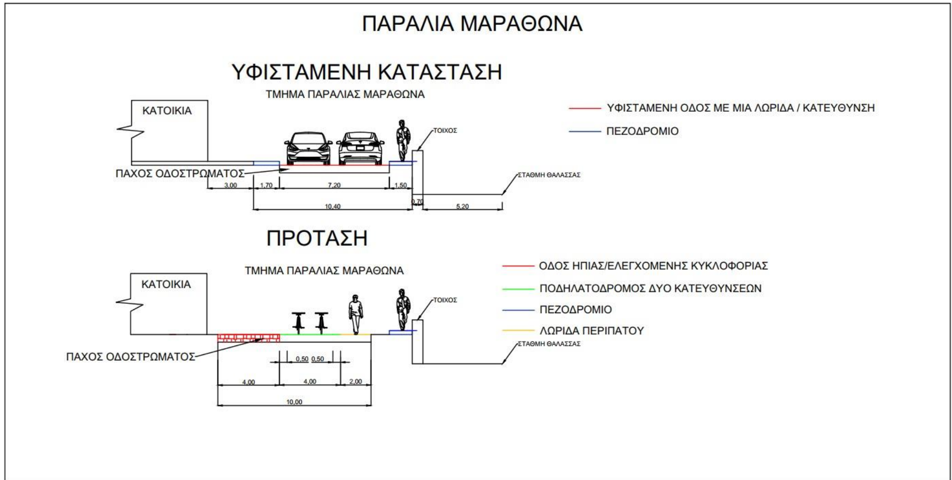
Εικόνα 9: Τυπική Διατομή στην Παραλία Μαραθώνα.
