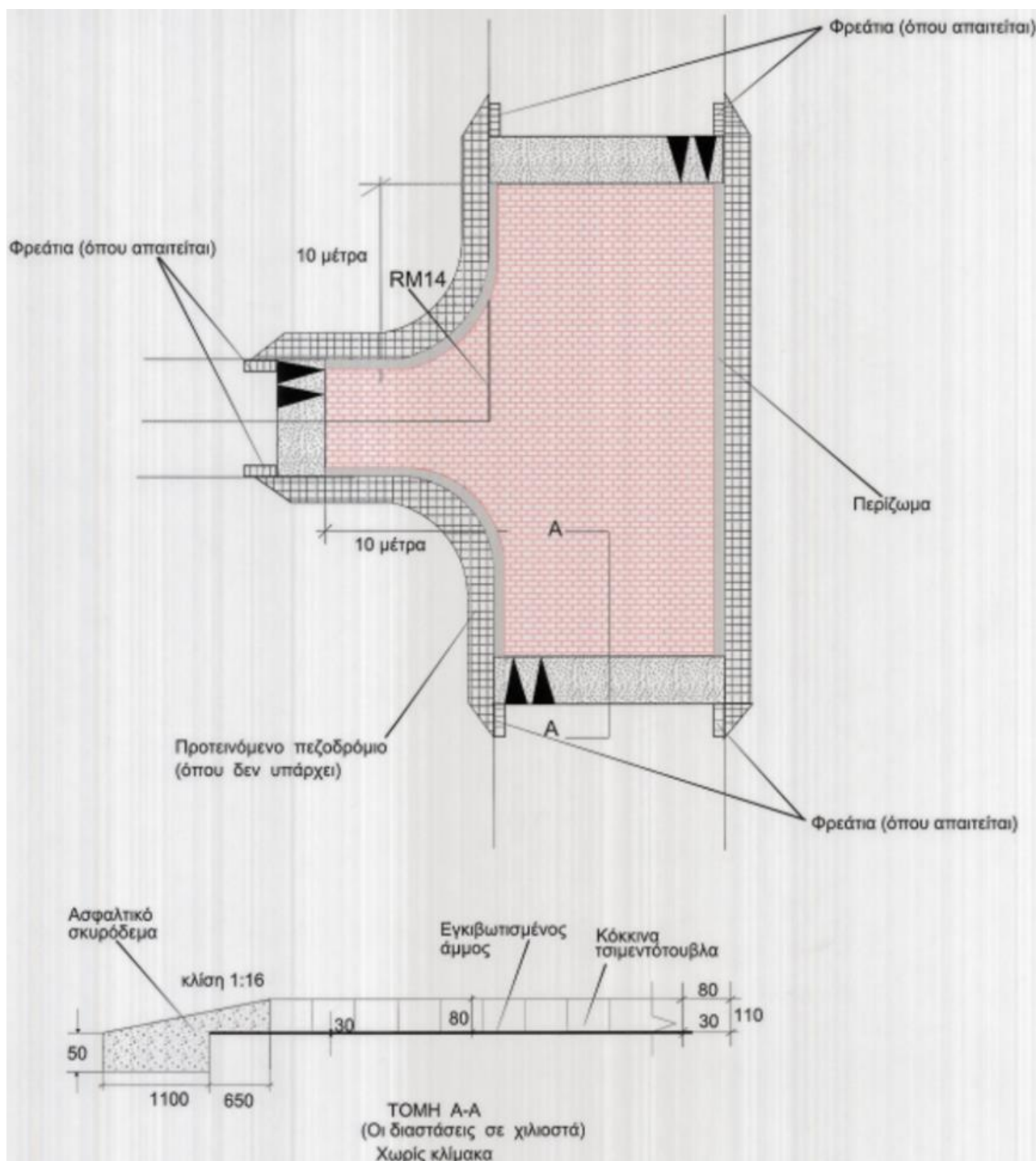
Εικόνα 17: Τυπικό Σχέδιο Υπερυψωμένης Συμβολής (πλατό).
